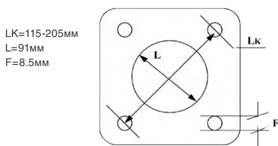
Рис.1 Фланцевое уплотнение
