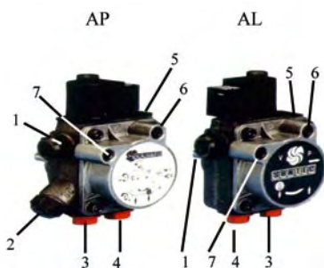
Рис.2 Топливный насос
