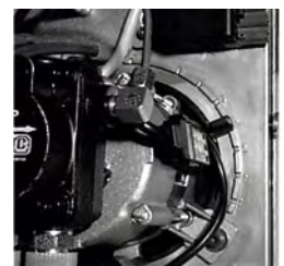
Рис.5 Дросельная заслонка
