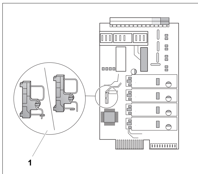
Рис. 12 Проволочная перемычка (например, у FM457)
