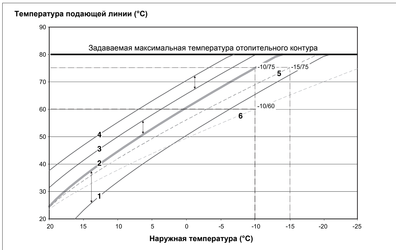
Рис. 21 Отопительная кривая для отопительной системы "Отопительный прибор"
