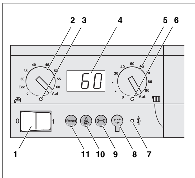
Рис. 14 Элементы управления BC10
