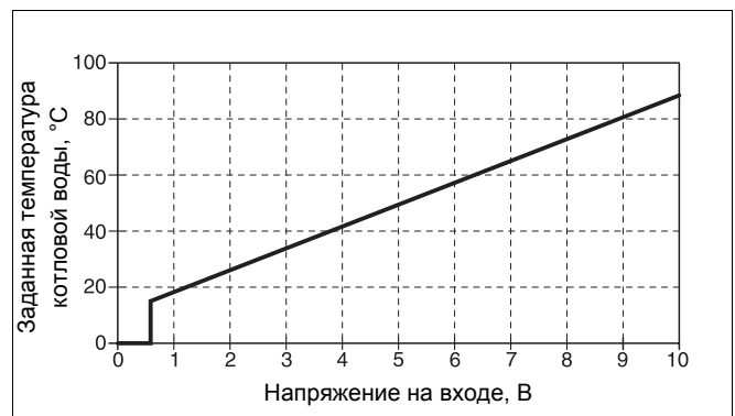
Рис. 11 Вход 0 – 10 В
